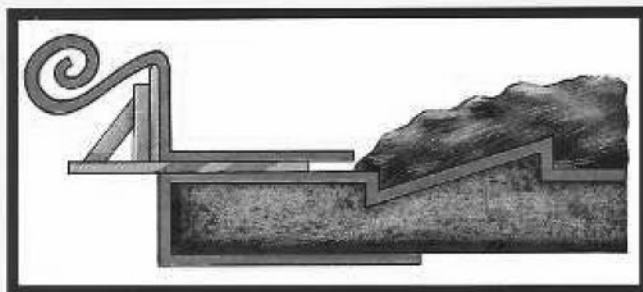
Przętawienie szalunku
